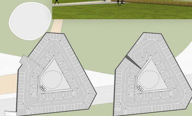
pianta parcheggi sotterranei 1:400
