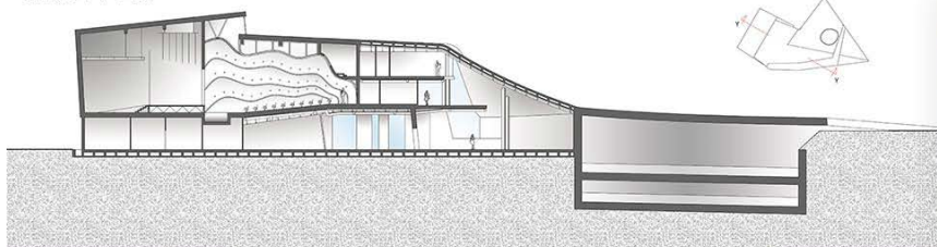
sezione Y-Y 1:200
